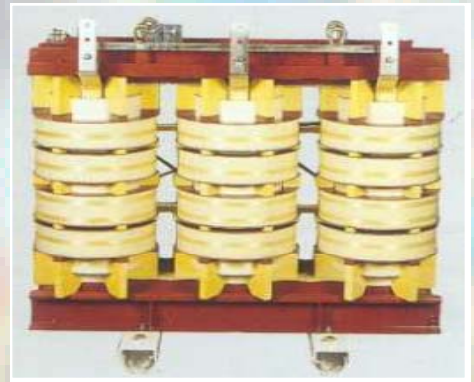
Transformateur de distribution sec Primaire: 20 000V - Secondaire: 410V Puissance: 630 kVA
